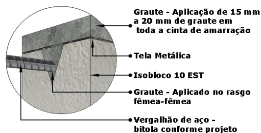
Detalhe Encunhamento
